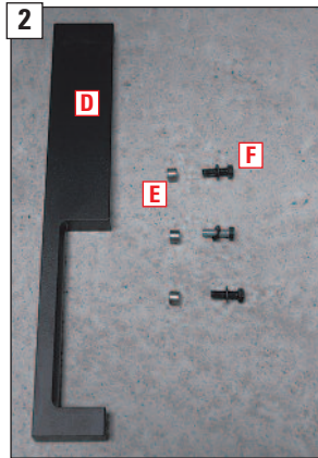
2 Detailansicht der werkseitigen Türgriffbefestigung.
