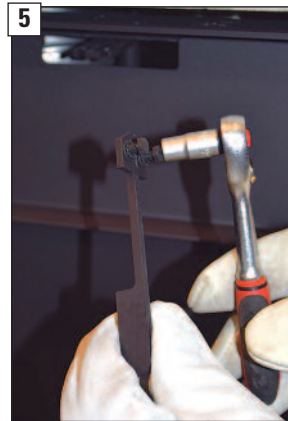
5 Befestigungsschrauben zur Montage soweit als möglich herausschrauben.
